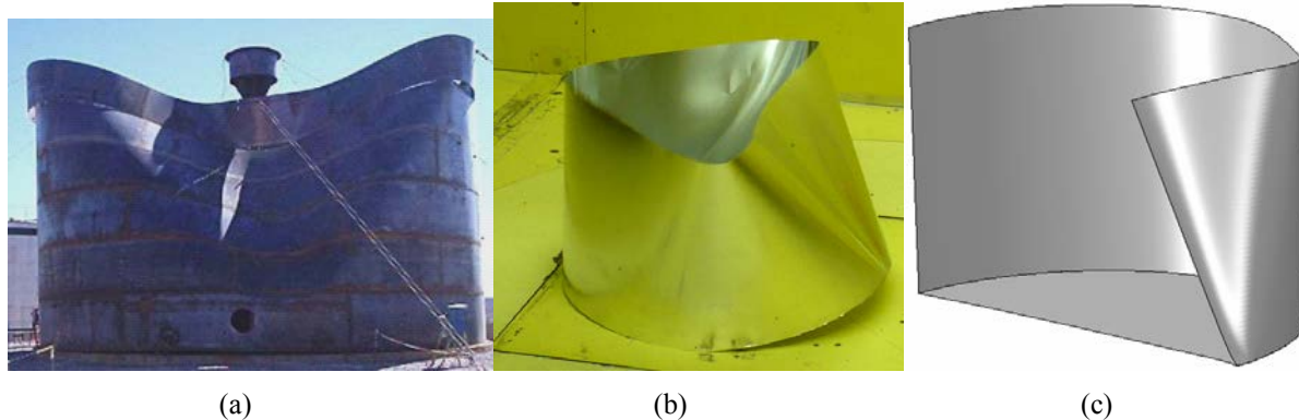
Figura 11: Comparación de deformadas, (a) tanque colapsado, (b) modelo ensayado, (c) modelo numérico.
