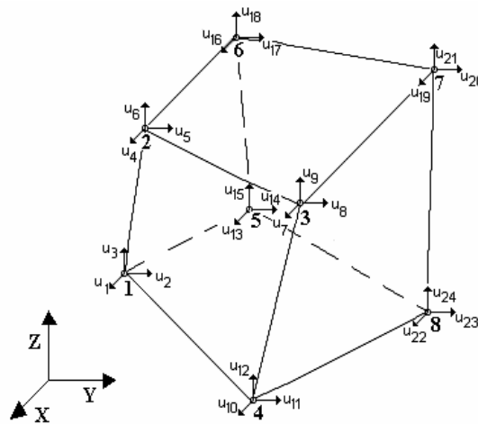
Figura 1. Configuración de nodos y grados de libertad por nodo
