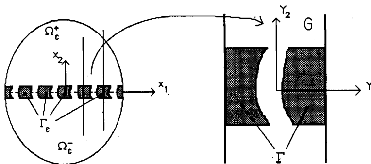
Figura 3. El dominio \Omega_\epsilon y el obstáculo \Gamma .
