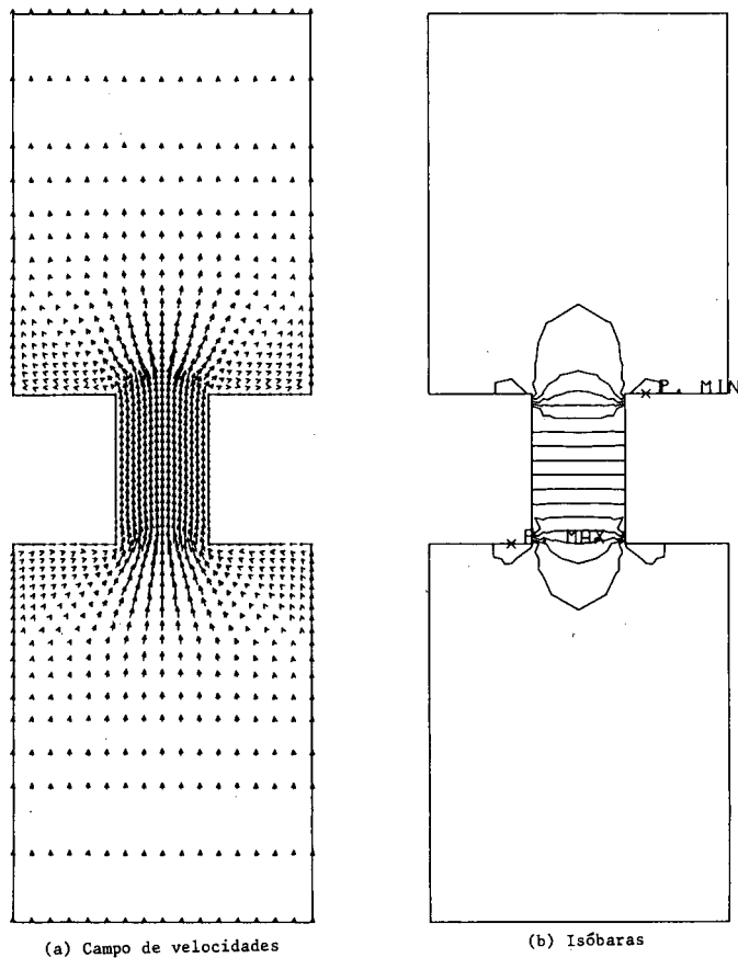
Figura 6. Resolución numérica del Problema Test N°1.
