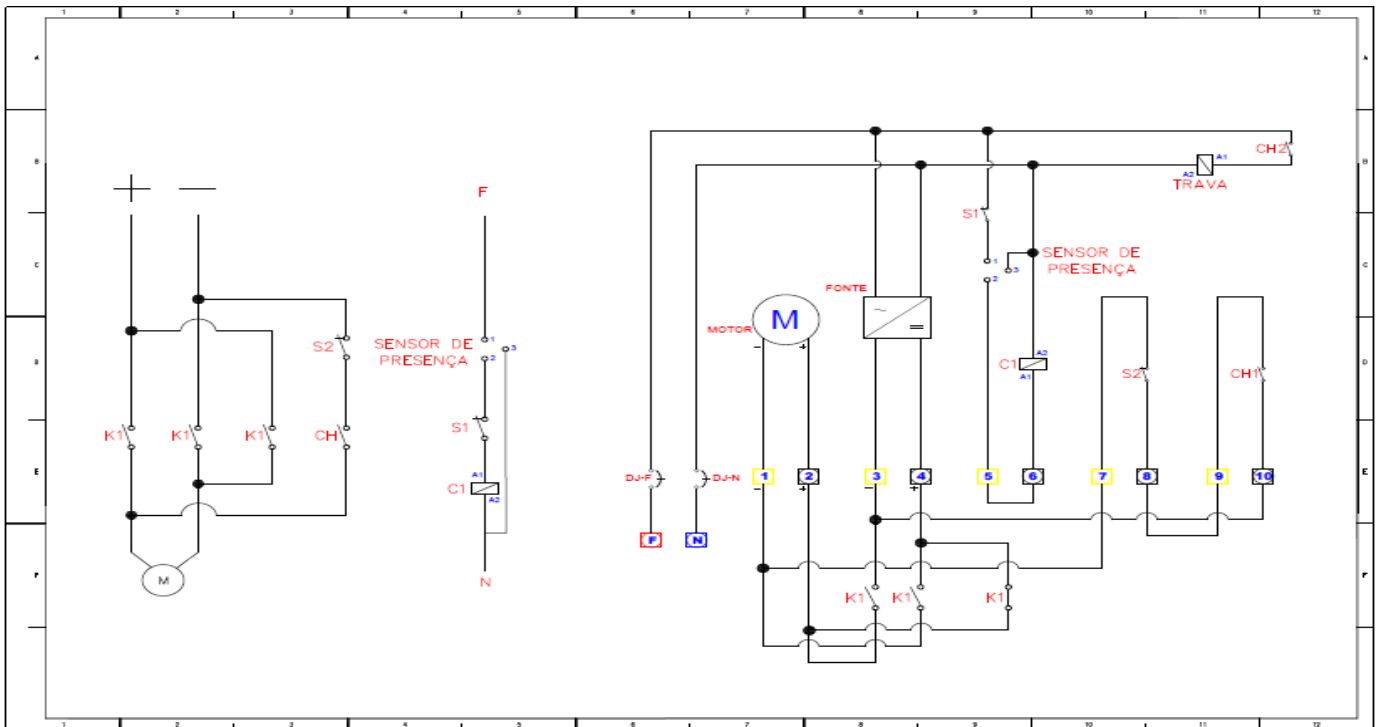
Figura 1. Diagrama Elétrico
