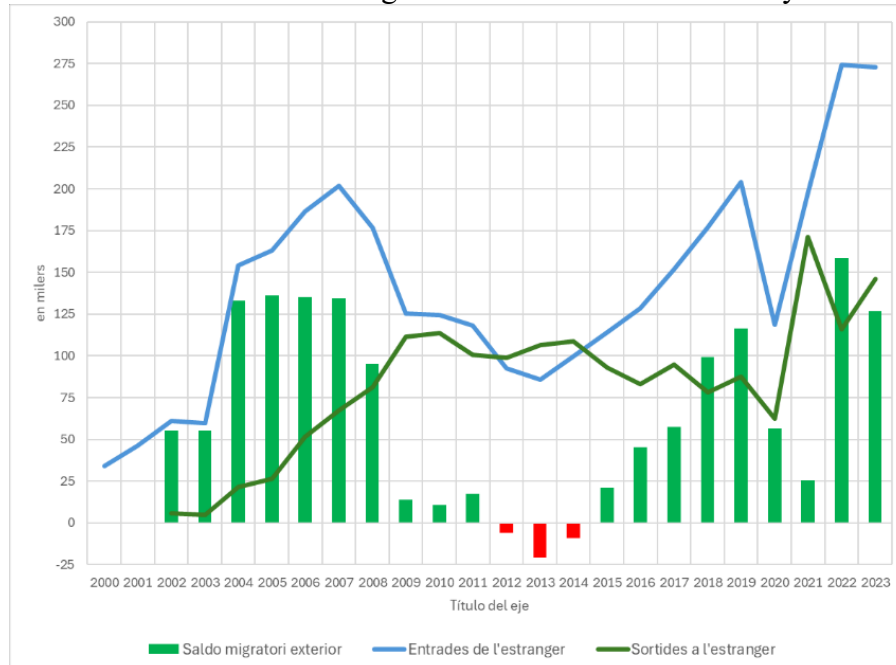
Figura 1: Evolució dels fluxos migratoris internacionals. Catalunya 2000-2023.
