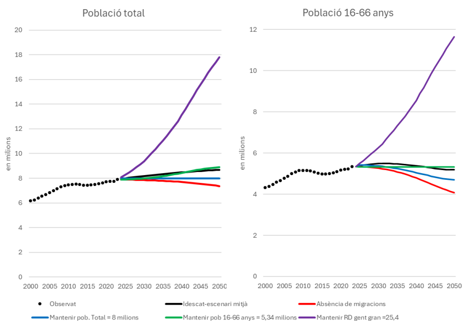
Figura 5: Evolució i projecció de la població de Catalunya 2000-2050 sota diferents supòsits.
