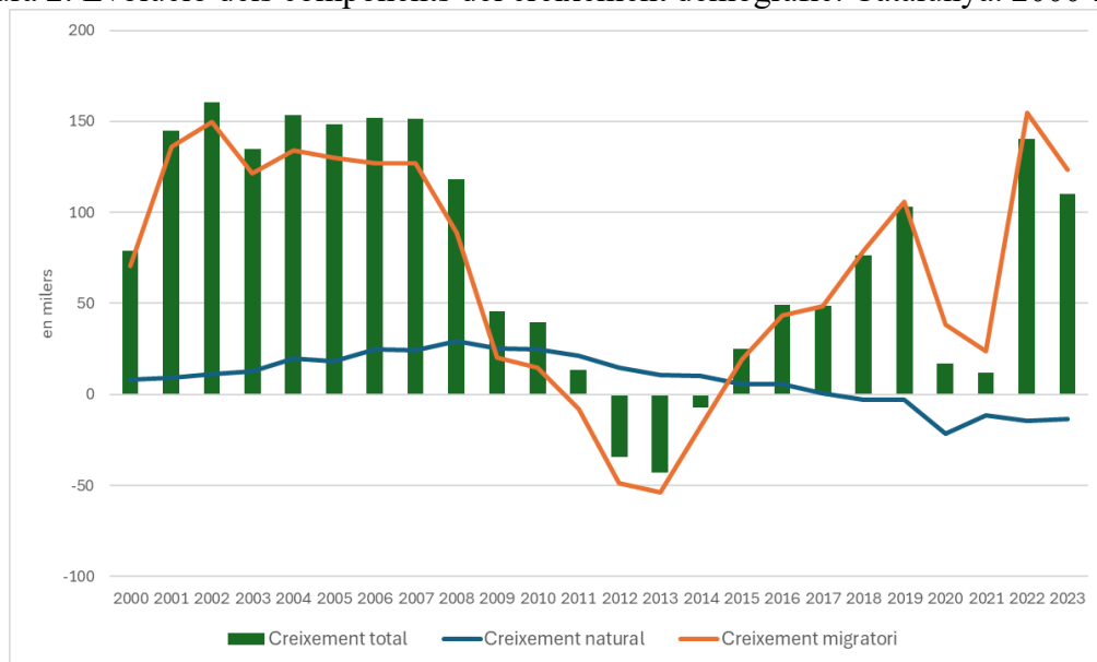
Figura 2: Evolució dels components del creixement demogràfic. Catalunya. 2000-2023.
