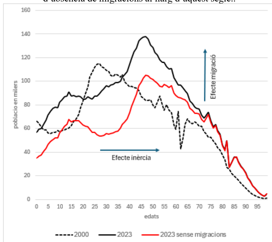
Figura 3: Estimació de la població de Catalunya a 1 de gener de 2023 sota el supòsit d'absència de migracions al llarg d'aquest segle..
