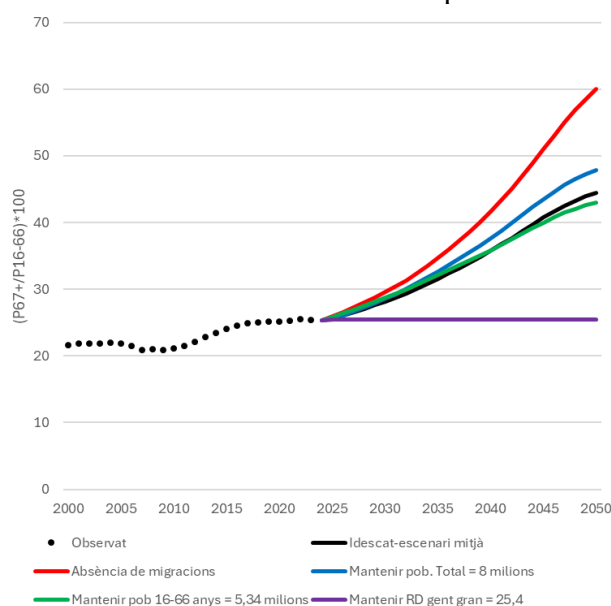
Figura 6: Evolució i projecció de la Relació de dependència de la gent gran a Catalunya 2000-2050 sota diferents supòsits.
