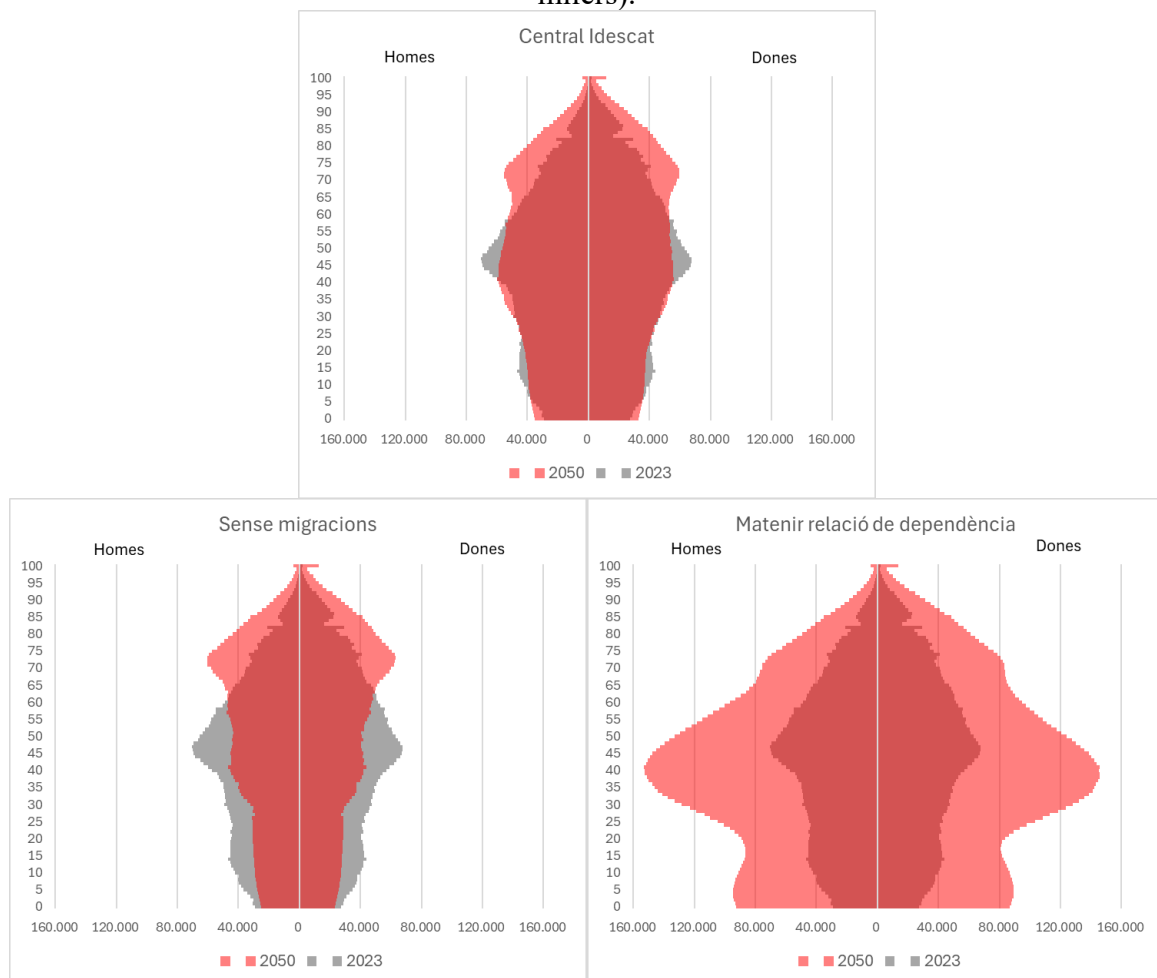
Figura 8: Piràmides de població de Catalunya 2023 i 2050 sota diferents supòsits (en milers).
