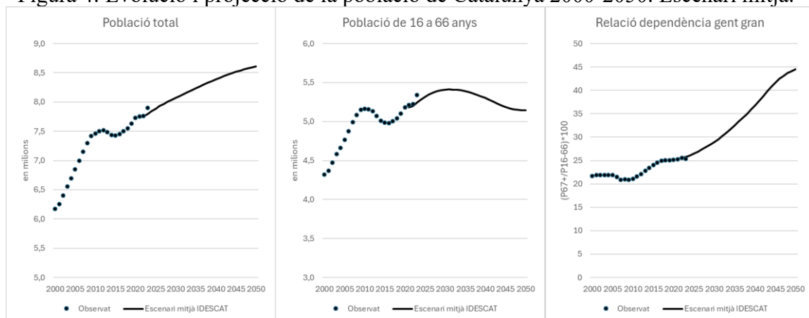
Figura 4: Evolució i projecció de la població de Catalunya 2000-2050. Escenari mitjà.
