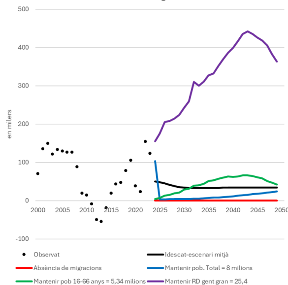
Figura 7: Evolució i projecció del saldo migratori de Catalunya 2000-2049 sota diferents supòsits.
