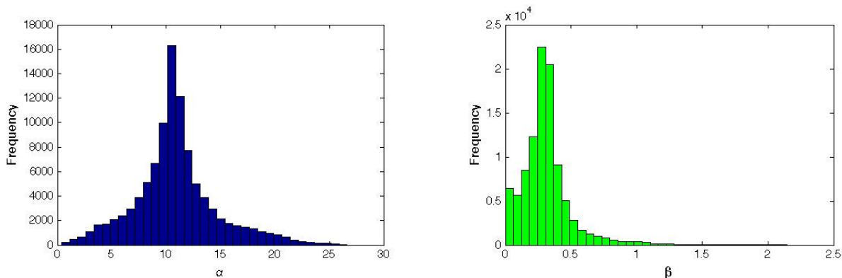
Figura 6: Distribuciones de frecuencia para el parámetro \alpha (a) y \beta (b).
