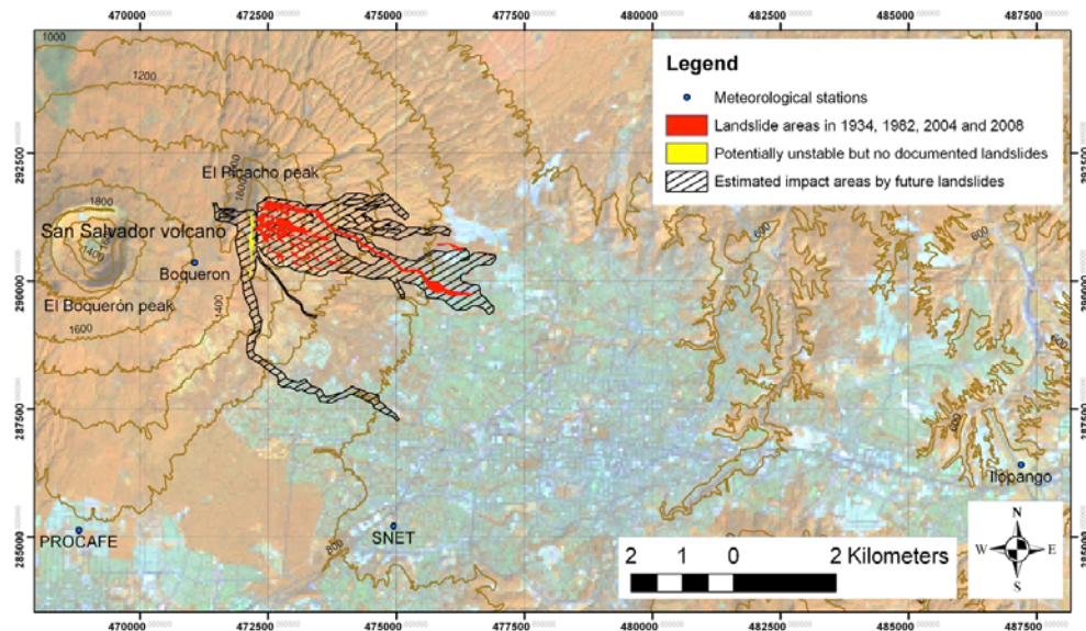
Figura 3: Pico el Picacho y áreas vecinas, incluyendo estaciones meteorológicas (puntos), áreas de deslizamientos de tierra anteriores (polígonos en rojo), y áreas susceptibles de deslizamientos (polígonos en amarillo y rallados).
