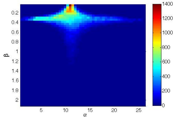
Figura 7: Mapa de frecuencias indicando la uni-modalidad de la distribución óptima de los parámetros del modelo, así como la estructura de correlación entre los parámetros del modelo.
