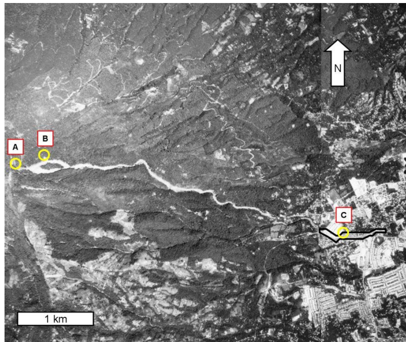
Figura 2: Foto aérea indicando el paso de la avalancha de flujo de lodos registrado en 1982: A) Corona de la zona de desgajamiento, B) marca de la media altura de la zona de ruptura, y C) zona de deposición.
