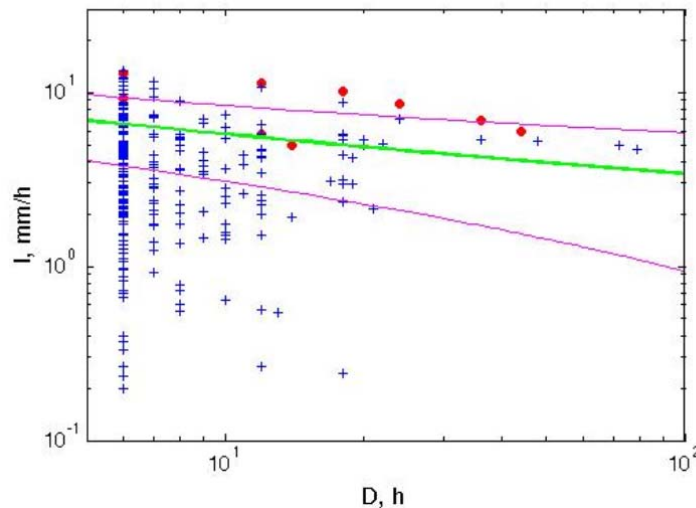
Figura 5: Base de datos utilizada para la clasificación probabilista, y definición del umbral medio y rango potencial de variación.
