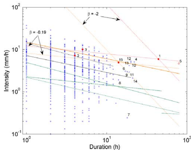
Figura 4: Datos de intensidad y duración para la estación El Boquerón, sobrepuestos con ecuaciones de umbrales propuestas predeterminados.
