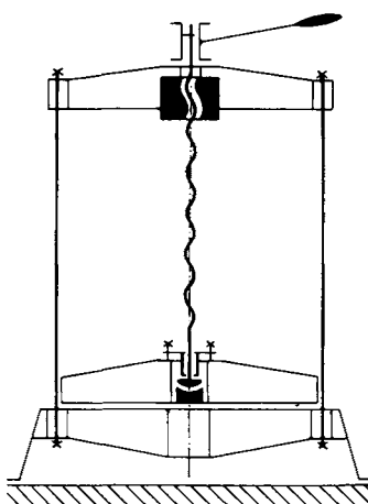
Figura 7. Diagrama cinemático de una prensa de tornillo.
