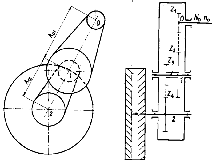
Figura 4. Diagrama cinemático de la caja de velocidades.
