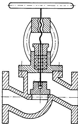
Figura 3. Diagrama cinemático de la válvula de asiento y cierre.
