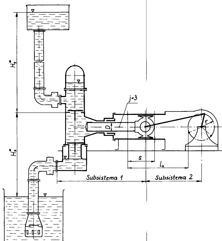
Figura 10. Diagrama cinemático de la bomba tricilíndrica de émbolo buzo.
