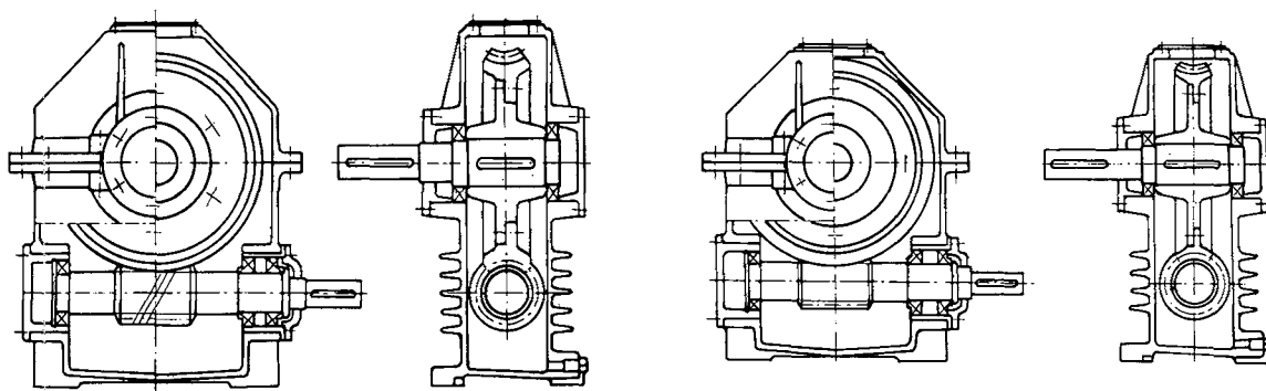
Figura 5. Engranaje de tornillo sin fin existente y óptimo.
