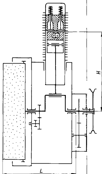
Figura 9. Diagrama cinemático del motor diesel monocilíndrico de un tractor.
