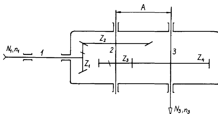
Figura 6. Diagrama cinemático del engranaje cónico/helicoidal de doble reducción.
