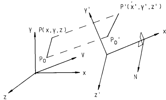
Figura 2. Proyección paralela.
