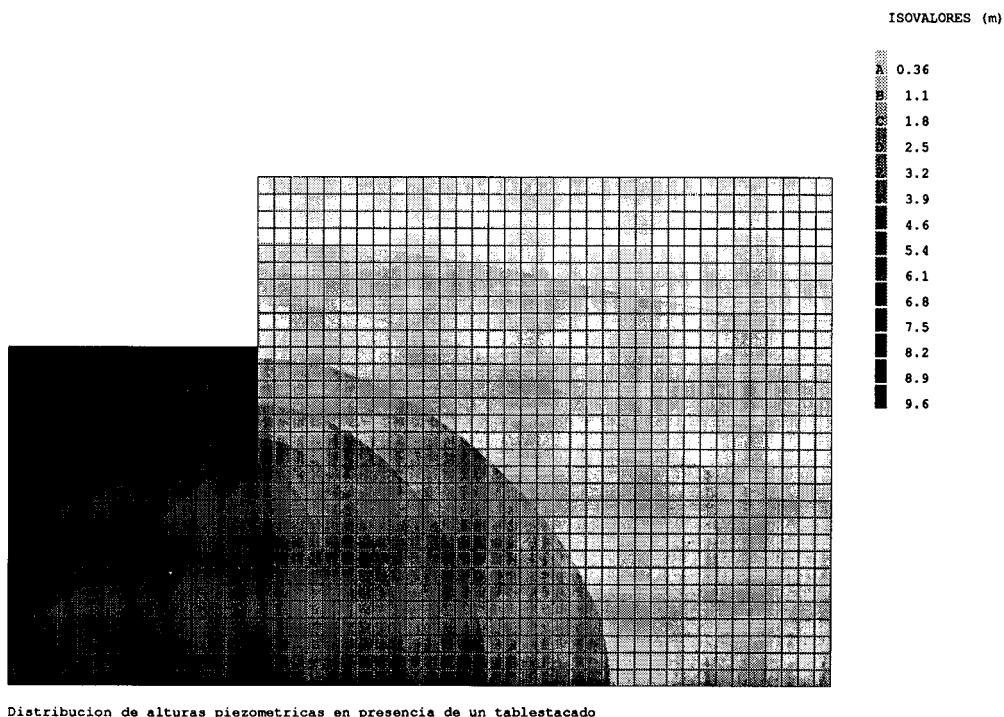
Distribucion de alturas piezometricas en presencia de un tablestacado
