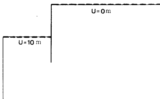
Figura 12. Filtración en medio poroso. Coeficiente de permeabilidad de 1 m/h en sentido horizontal. Condiciones de contorno y ley de alturas piezométricas (m), régimen estacionario
