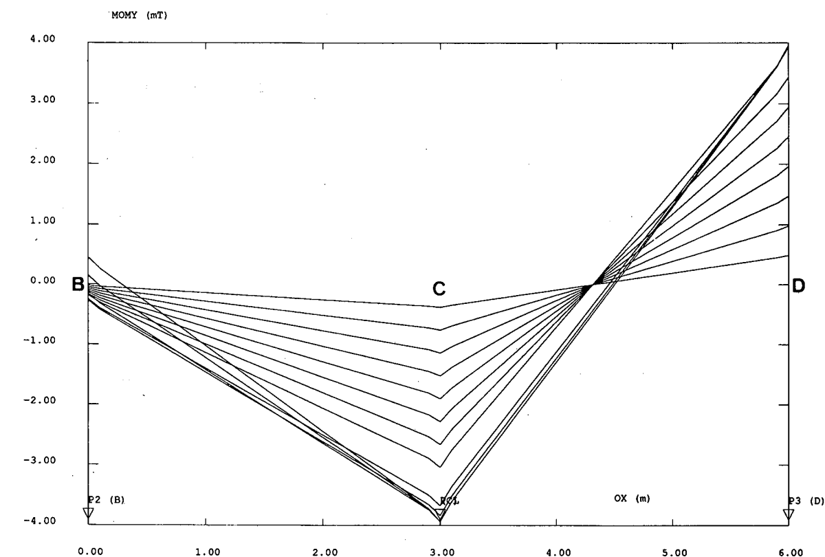
Evolucion del momento flector en el dintel
