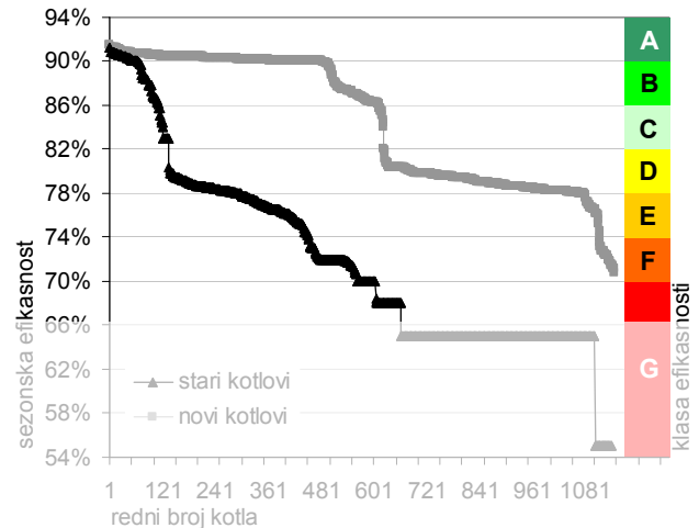
Слика 2: Приказ SEDBUK за преко 2000 котлова [6]
