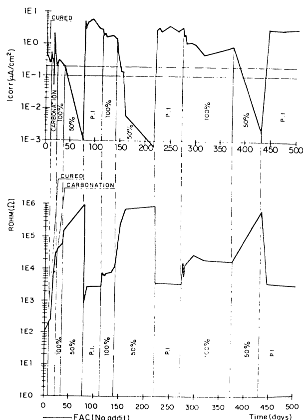
Fig. 4.—Intensidad de corrosión ( i_{corr} \mu A/cm^2 ) y caída óhmica ( R_{ohm} \Omega ) en función del tiempo para barras de acero embebidas en mortero de cemento de cenizas carbonatado.
