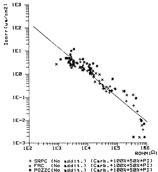
Fig. 6.—Intensidad de corrosión ( i_{corr} \mu\text{A}/\text{cm}^2 ) en función de la caída óhmica ( R_{ohm} \Omega ) para barras de acero embebidas en morteros carbonatados de cements.
