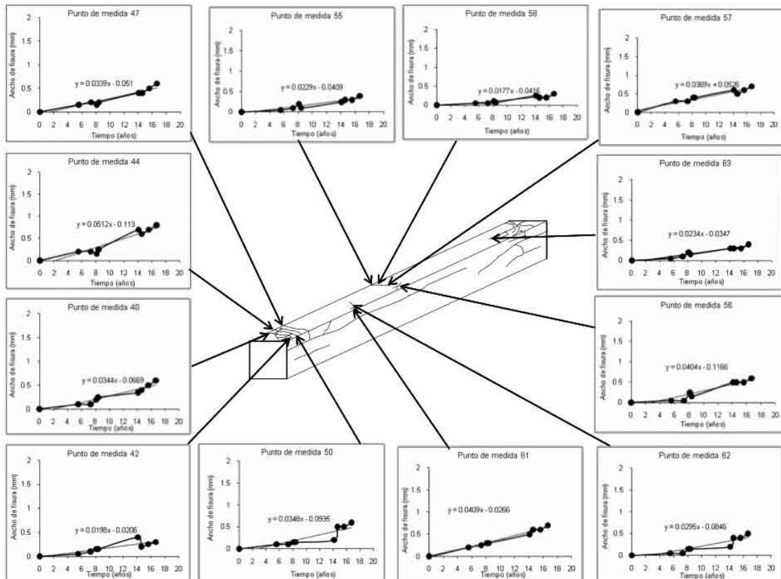
Fig. 4. Grietas en la columna y su seguimiento.
