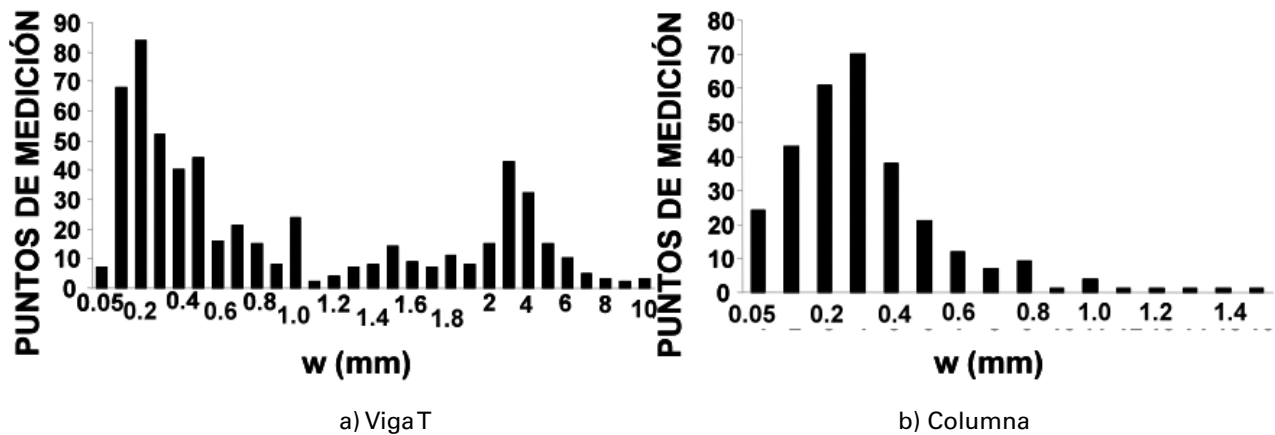
Fig. 7. Distribución de datos agrietamiento de viga T y columna (corrosión natural).
