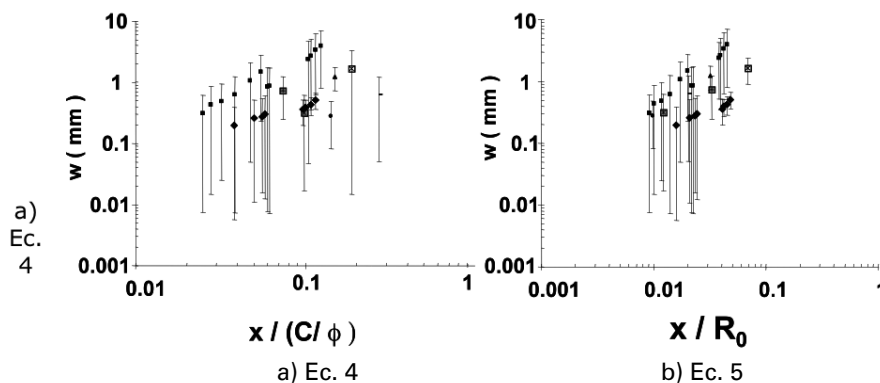
Fig. 6. Relación de agrietamiento de viga T, columna (corrosión natural) y otros investigadores (corrosión acelerada) con las ecuaciones propuestas. Dispersion de los datos, escala logarítmica.
