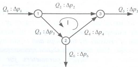
Slika 1: Segment prstenaste gasne mreže
