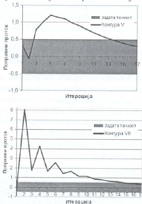
Slika 4 1 : Promene vrednosti popravnih protoka (u \text{m}^3/\text{h} ) za dve konture date mreže
