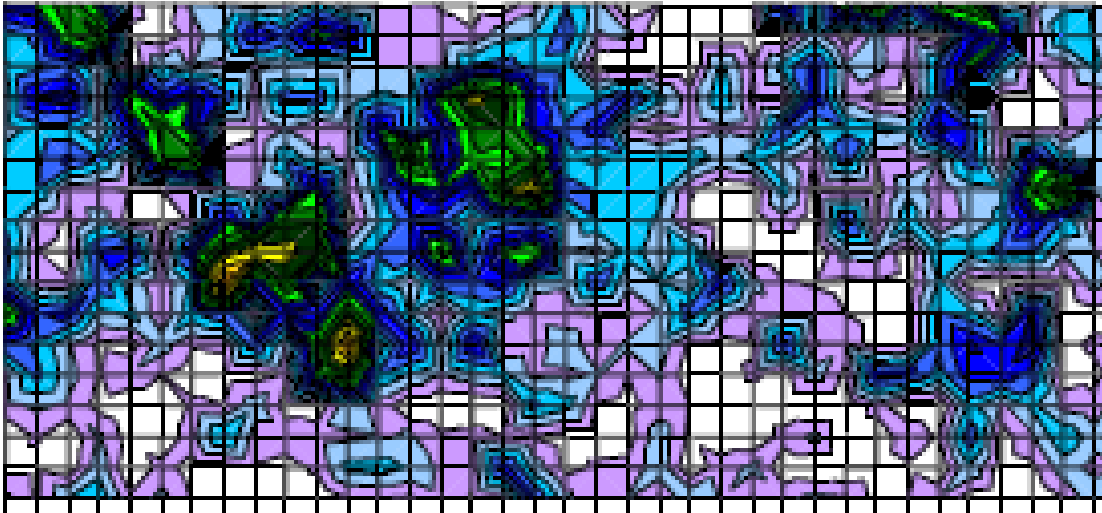
Figure 26: Actual Corrosion
