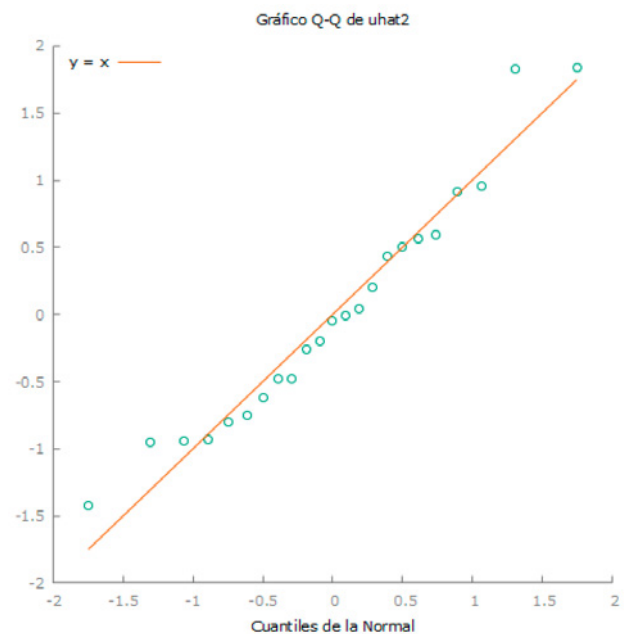
Il·lustració 24: Gràfic Q-Q del Model 1
