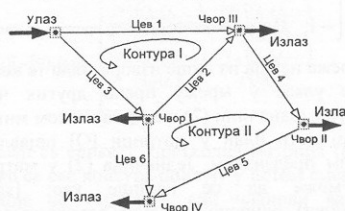
Слика 1: Гасна прстенаста дистрибутивна мрежа Прорачун мреже се даље врши тако да се као резултат прорачунају протоци кроз деонице у зависности од изабраног пречника цеви. На крају се врши провера дозвољених брзина струјања гаса по деоницама и
