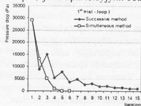
Слика 2: Падови притиска по итерацијама за једну контуру гасне мреже
