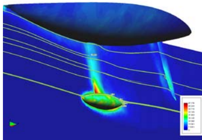
Cálculo hidrodinámico con TDYN del barco Bravo España (Copa América 1999)
