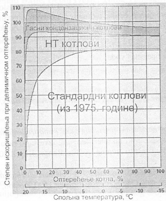
Slika 4. Dijagram zavisnosti stepena iskorišćenja od opterećenju kotla za tri različite vrste kotlova
