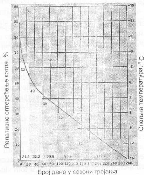
Slika 2. Dijagram za određivanje srednjeg stepena iskorišćenja prema DIN 4702-8
