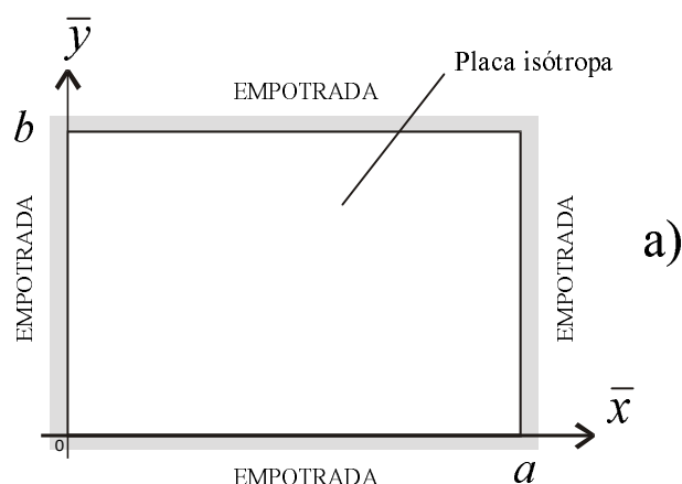
Figura 4a. Placa rectangular isótropa maciza, empotrada en los cuatro bordes con \lambda = 3/2
