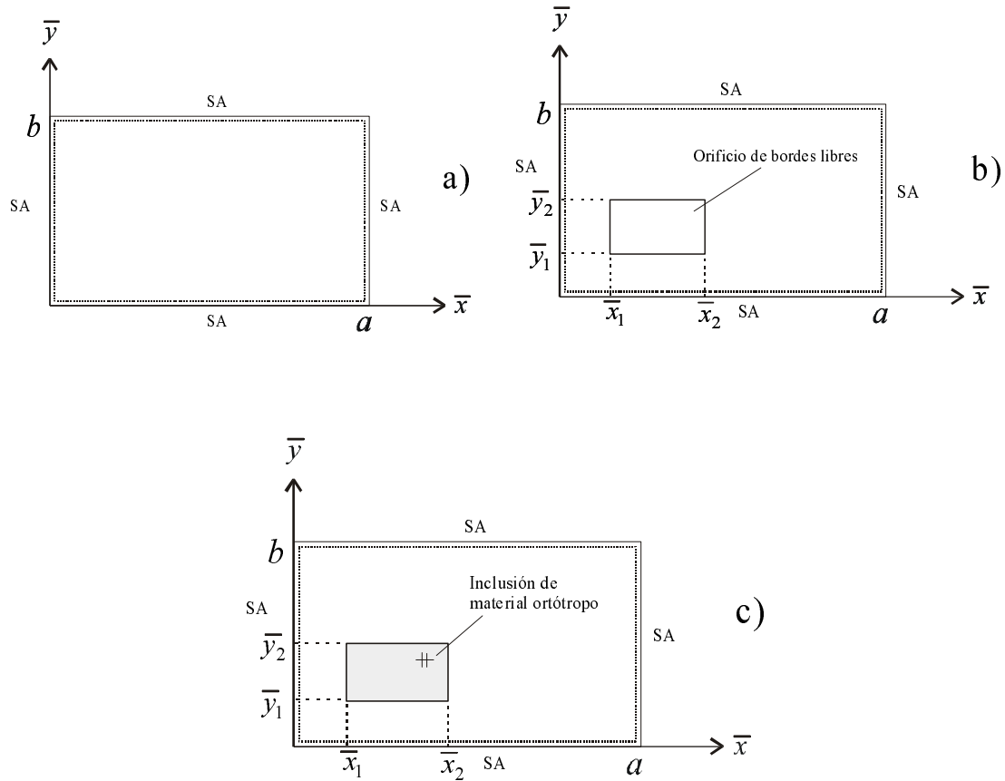
Figura 5. Placa rectangular isotrópica simplemente apoyada en su contorno: a) maciza, b) con un hueco, c) con una inclusión de material ortótropo D_{1inc}/D = 2,856 ; D_{2inc}/D = 2,256 ; \nu_{2inc} = 0,757 ; D_{kinc}/D = 0,765 y \rho_{inc}/\rho = 2,95
