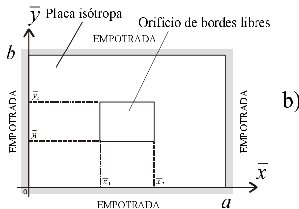
Figura 4b. Placa rectangular isótropa con un hueco de igual relación de lados \lambda y de dimensiones (x_2 - x_1) \times (y_2 - y_1) , empotrada en los cuatro bordes con \lambda = 3/2
