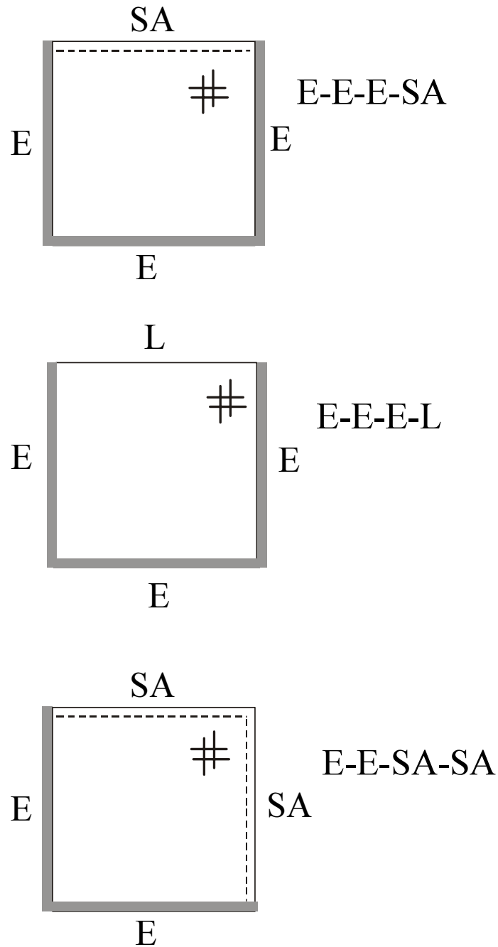
Figura 6. Placa rectangular ortótropa maciza con diferentes condiciones de borde D_2/D_1 = 1/2 ; D_k/D_1 = 1/2 y \nu_2 = 0,3
