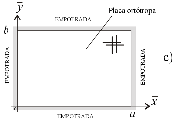
Figura 4c. Placa rectangular ortótropa maciza, D_2 = D_1/2 ; \nu_2 = 0,30 ; D_k = D_1/2 , empotrada en los cuatro bordes con \lambda = 3/2
