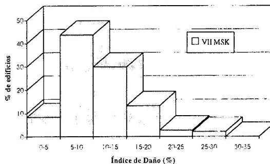
Figura 19. Histograma de frecuencias del índice de daño para I=VII
