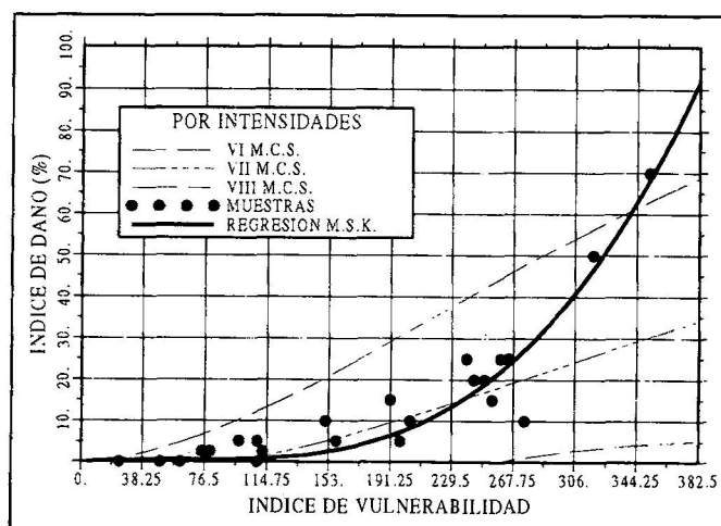
Figura 1. Función de vulnerabilidad observada en España, para un nivel de intensidad VII MSK 2 . En trazos entrecortados se representan las funciones propuestas por Angeletti et al. 6
