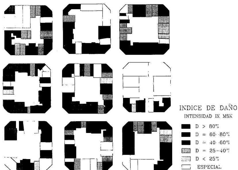
Figura 17. Escenario de daño para un sismo de intensidad IX MSK
