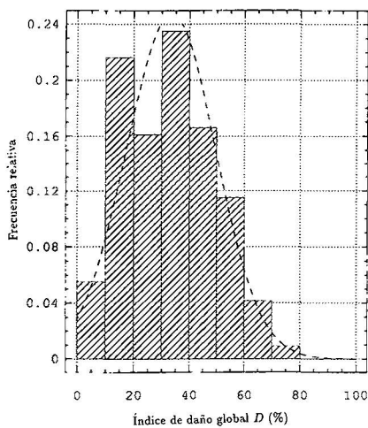
Figura 11. Histograma y distribución normal del daño. I_v \in [250,300] , I=VII MSK
