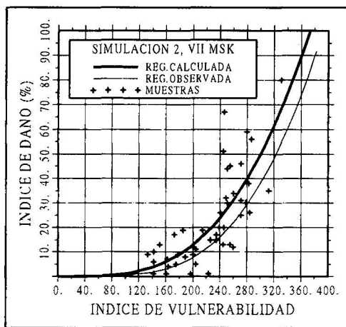
Figura 4. Segunda simulación para intensidad VII y comparación con la función observada
