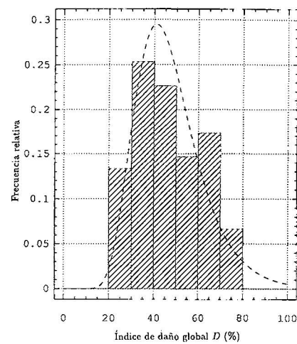
Figura 12. Histograma y distribución normal del daño. I_v \in [300,350] , I=VII MSK
