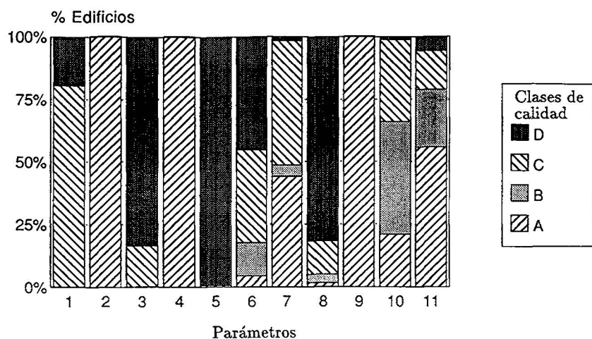
Figura 22. Parámetros que constituyen la vulnerabilidad de la muestra
