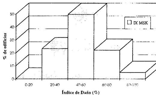
Figura 21. Histograma de frecuencias del índice de daño para I=IX
