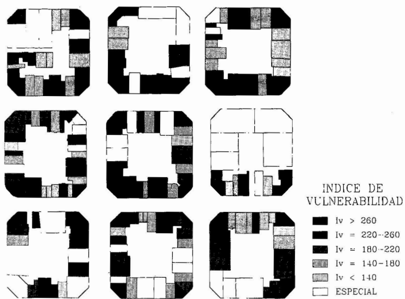
Figura 14. Mapa de vulnerabilidad del sector estudiado
