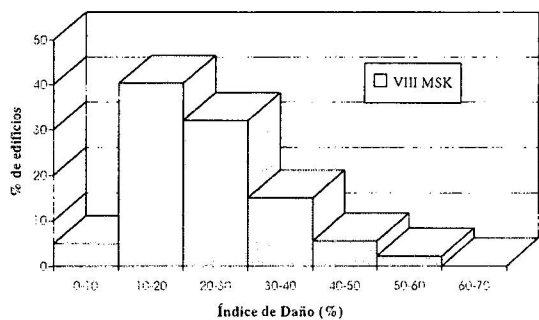
Figura 20. Histograma de frecuencias del índice de daño para I=VIII
