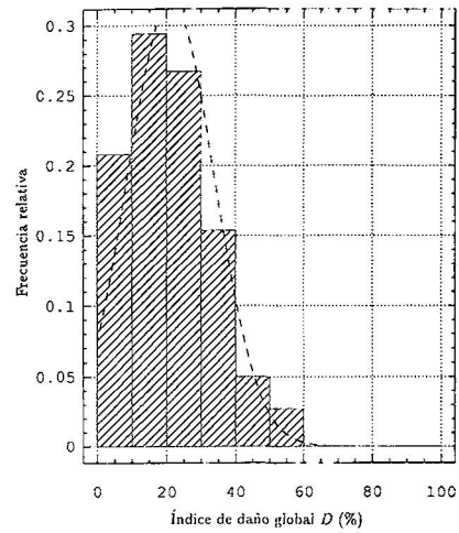
Figura 10. Histograma y distribución normal del daño. I_v \in [200,250] , I=VII MSK
