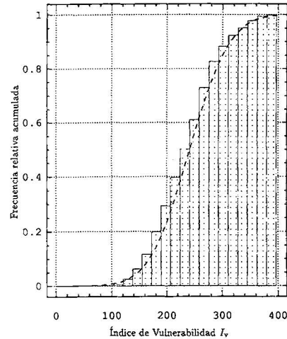
Figura 8. Frecuencias acumuladas y ajuste a la función de distribución normal para el índice de vulnerabilidad
