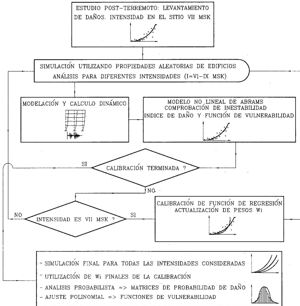
Figura 2. Algoritmo general del proceso de simulación
