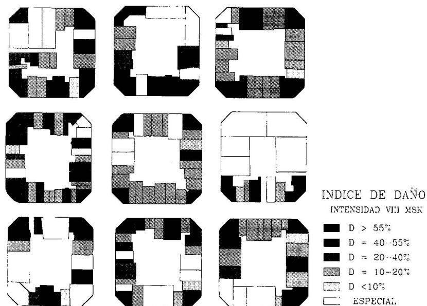
Figura 16. Escenario de daño para un sismo de intensidad VIII MSK
