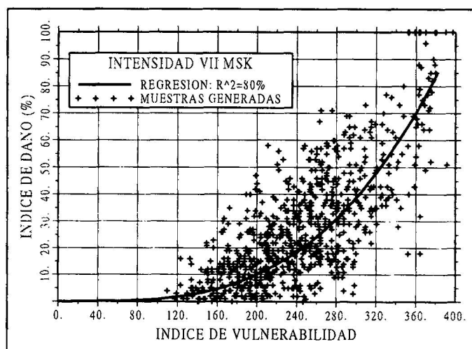
Figura 6. Simulación final de edificios y regresión polinómica para intensidad VII MSK
