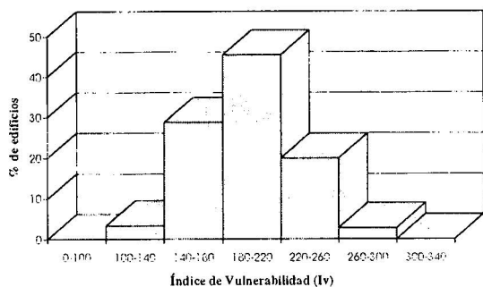
Figura 18. Histograma de frecuencias del índice de vulnerabilidad
