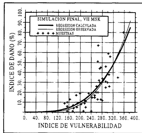
Figura 5. Simulación final de edificios para intensidad VII y comparación con la función observada
