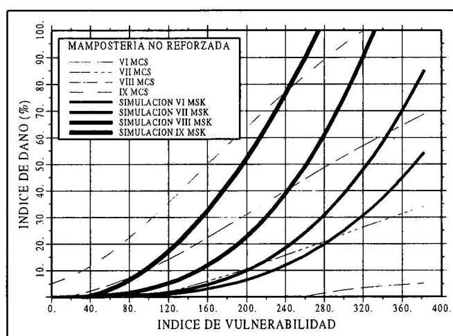
Figura 13. Funciones de vulnerabilidad obtenidas por simulación para mampostería no reforzada y diferentes escalas de intensidad MSK. Las líneas discontinuas representan las curvas italianas propuestas en la referencia 6
