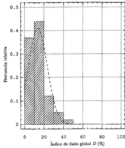
Figura 9. Histograma y distribución normal del daño. I_v \in [150,200] , I=VII MSK
