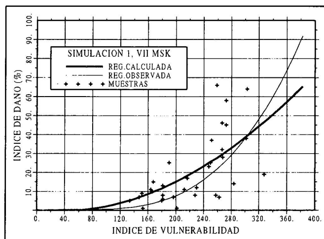
Figura 3. Primera simulación de edificios para intensidad VII y comparación con la función observada
