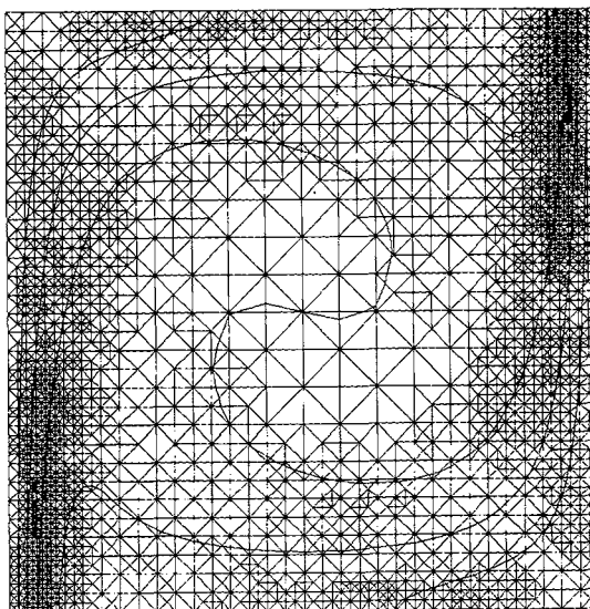
Figura 6(a). Indicador 1, 3022 nodos, 4 refinamientos.
